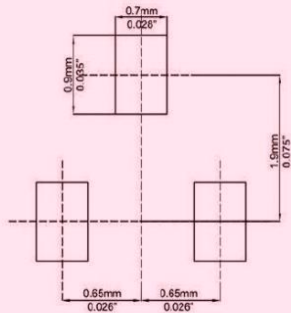
SOT-323
